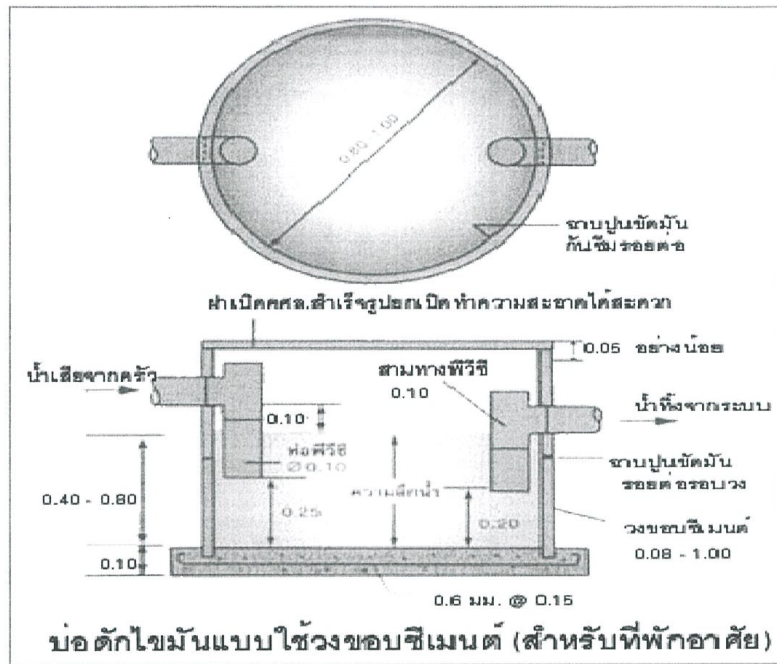
ขนาดมาตรฐานบ่อดักไขมันแบบวงขอบซีเมนต์สำหรับบ้านพักอาศัย
